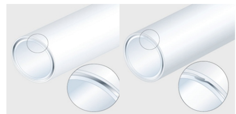
搭接焊多层复合管 需更厚塑料层以保证壁厚均匀
